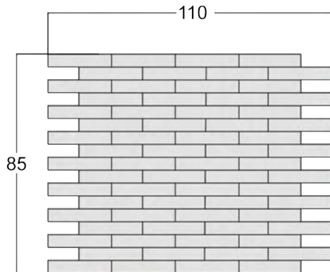
Forma y medidas
